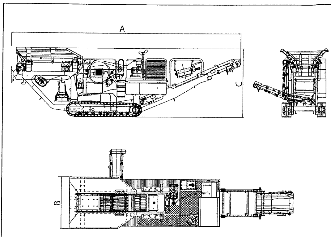
Abbildung 3-1 LT96 in Betriebsposition
