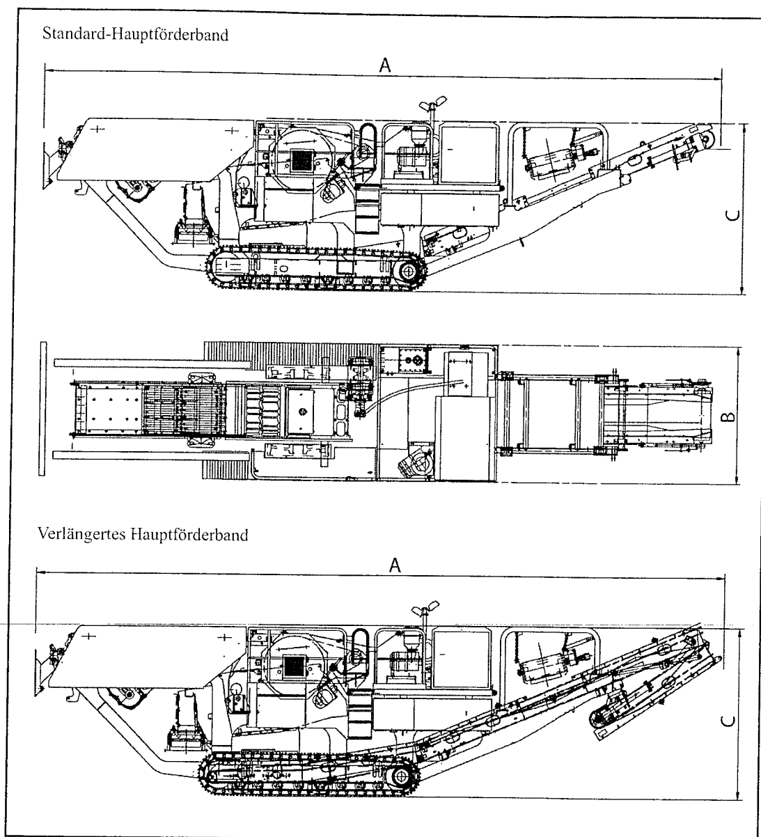
Abbildung 3-2 LT116 in Transportposition
